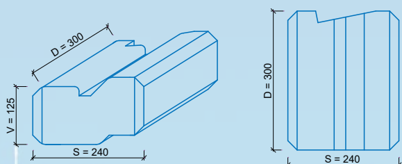
Obr. 1. Schéma betónovej tvárnice
